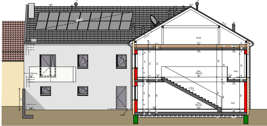
Ansicht Süd & Schnitt A-A
