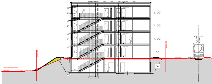
SCHNITT A-A
