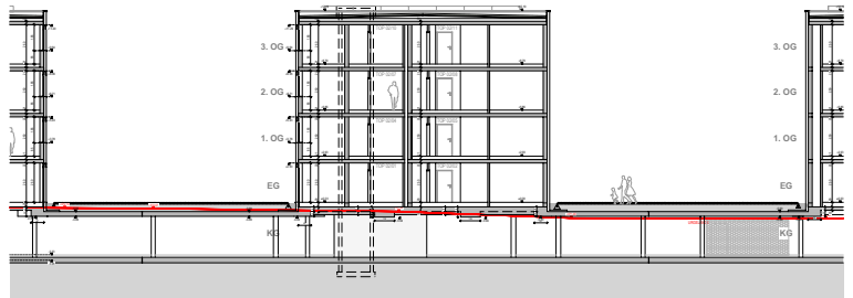
SCHNITT B-B
