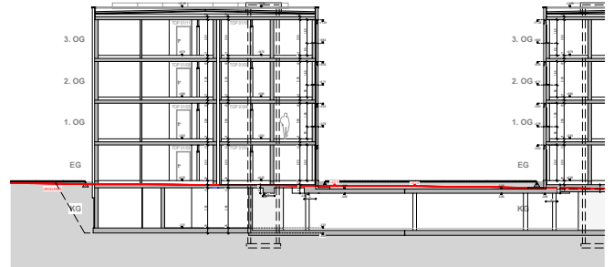
SCHNITT B-B
