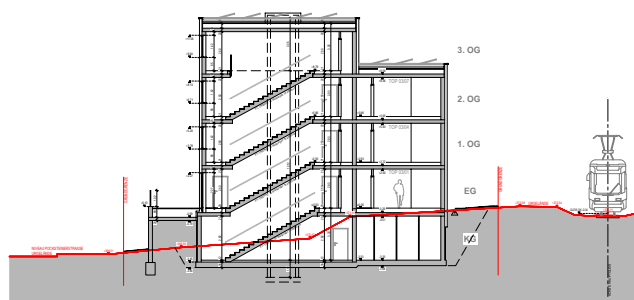
SCHNITT A-A
