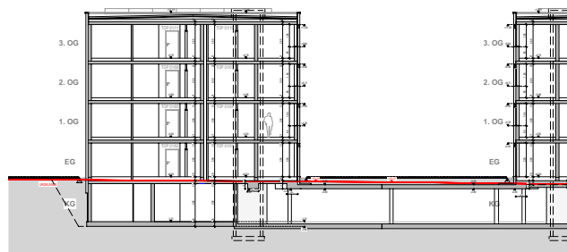
SCHNITT B-B
