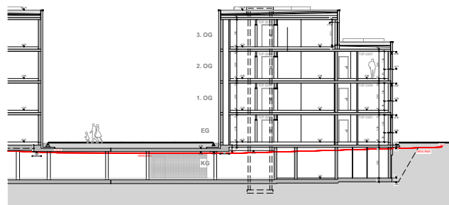
SCHNITT B-B
