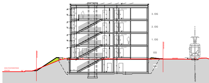
SCHNITT A-A
