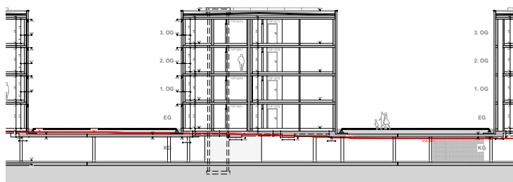
SCHNITT B-B
