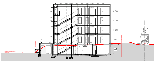
SCHNITT A-A
